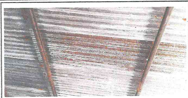
Foto1: Oxido en lámina y costanera
